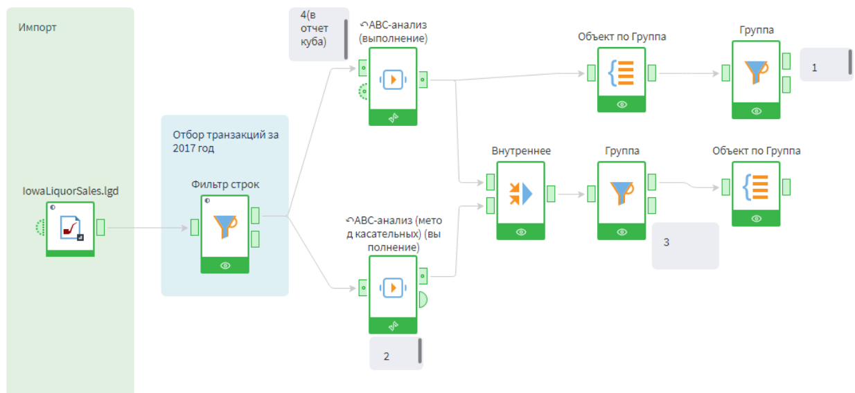
Рисунок 7 – Схема для многомерного ABC-анализа
