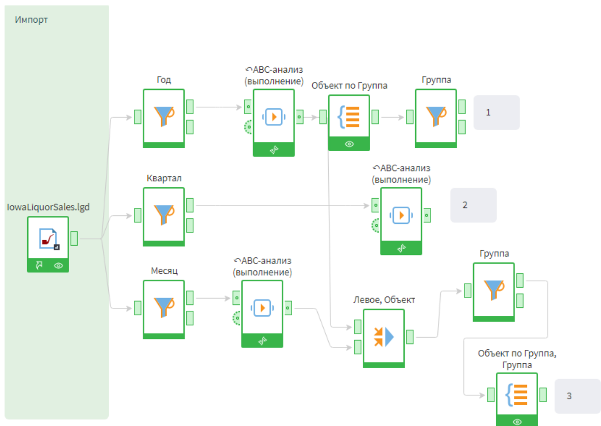
Рисунок 11 – Схема для ABC-анализа по периодам
