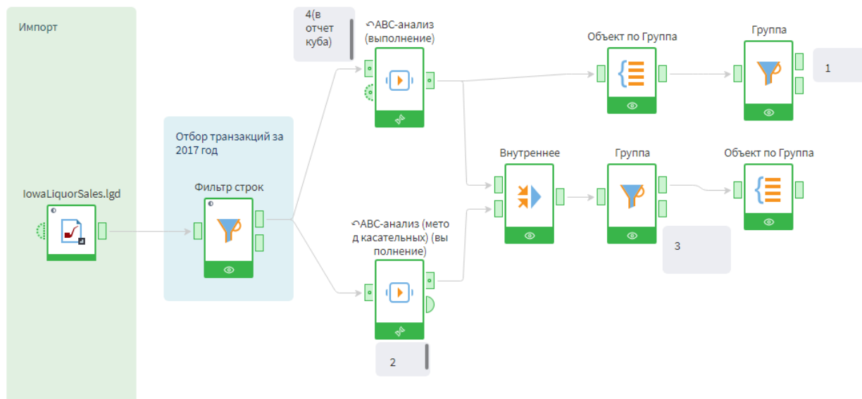
Рисунок 2 – Схема для классического ABC-анализа
