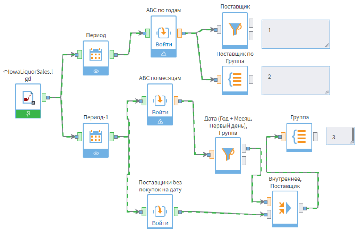
Рисунок 15 – Схема для ABC-анализа в динамике
